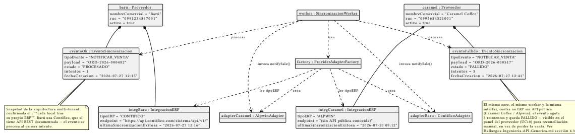
Figure 4: Diagrama de objetos: integración ERP
